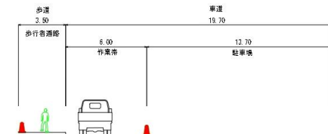
A-A' 断面図 S = 1 : 250
